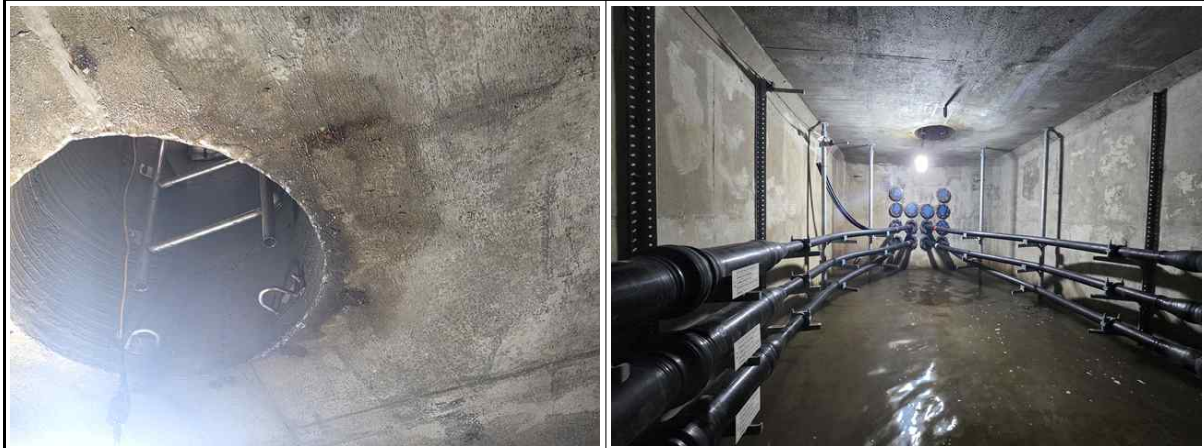
【사진 1.22】 맨홀 내부 주요 손상
